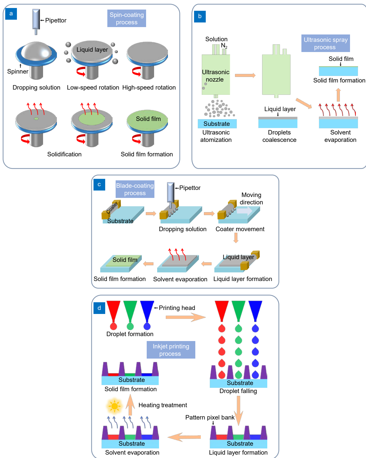
图 4 湿法工艺示意图。
